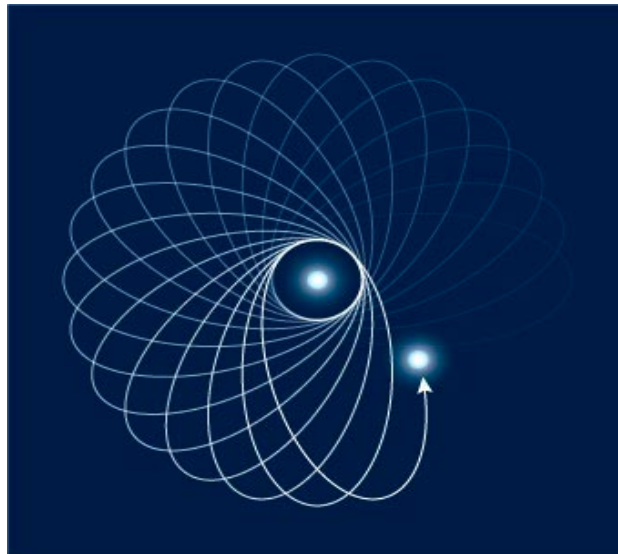
شکل ۴: تصویر بسیار اغراق آمیزی از حرکت تقدیمی عطارد
